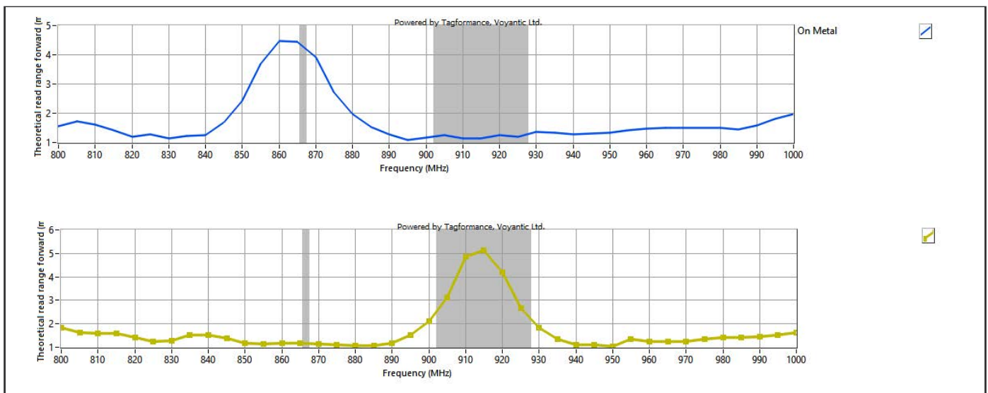
UNI 6006- RF performance(M730)
